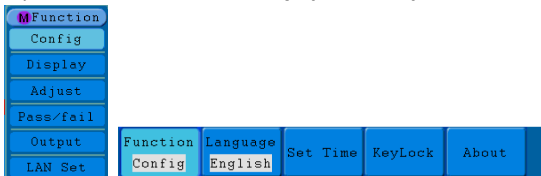
Fig. 52 Configuration Menu
