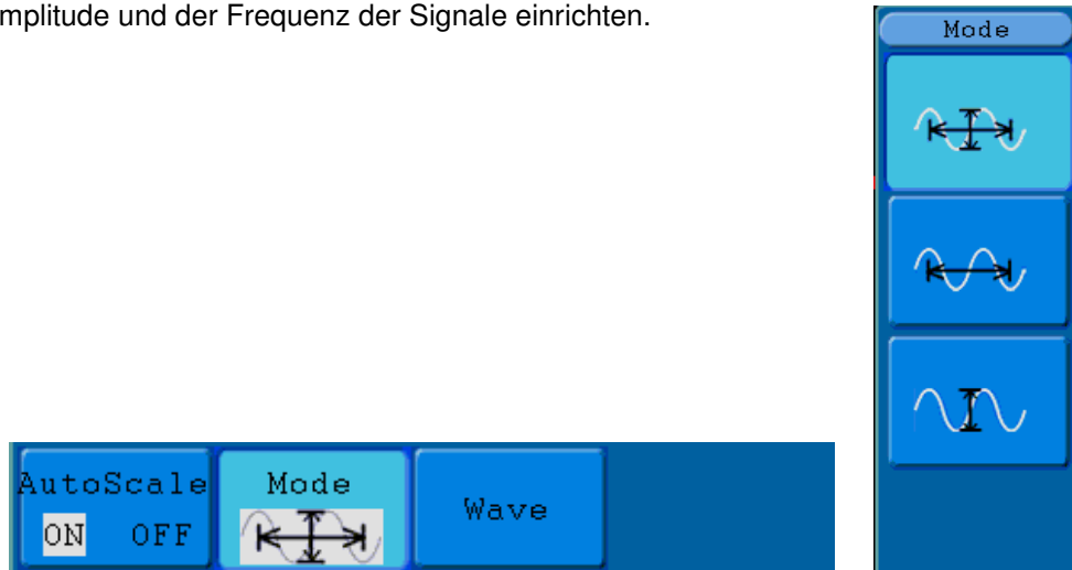
Abb. 76 Autoscale-Menü
