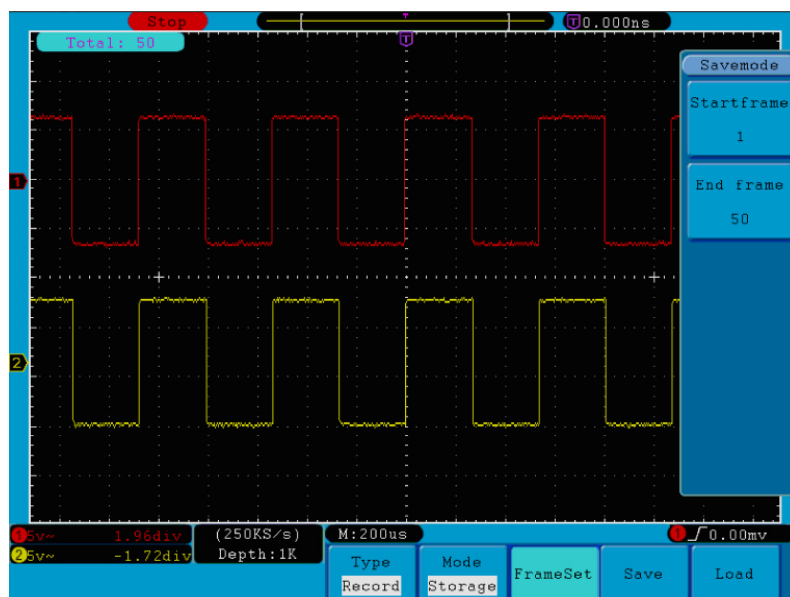
Abb.51 Wellenform-Speicherung
