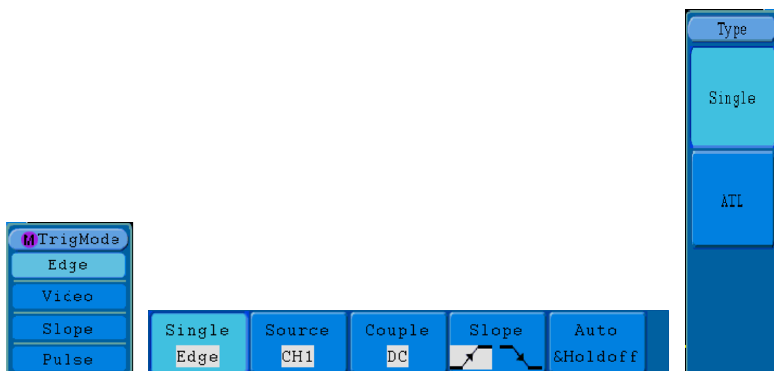
Fig. 30 Edge trigger menu
